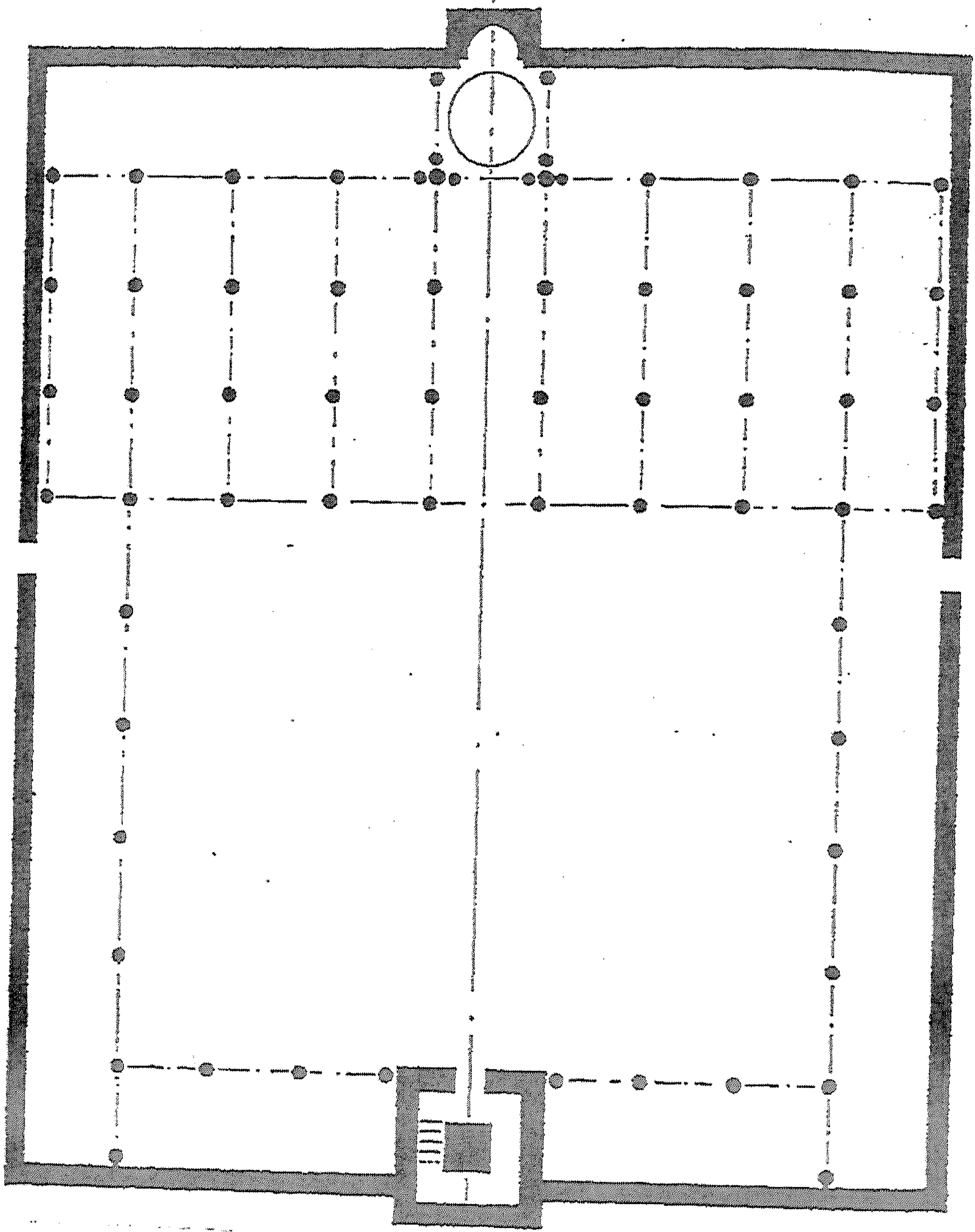
(شكل رقم ٤٠) رسم تخطيطي لجامع صفاقس في عهد الأغلبية عن ليزين
